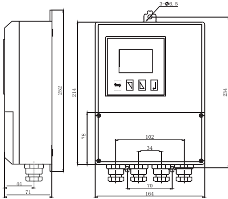
分体式转换器尺寸
