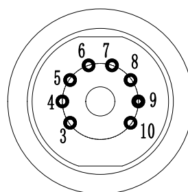
压力 - 温度信号输出
